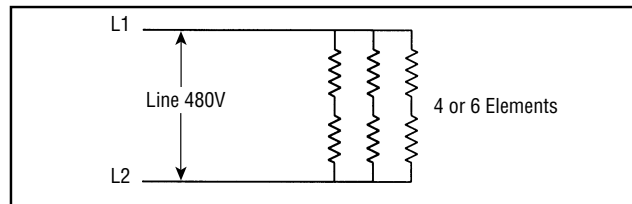
Figure 2 — 480 Volt Heaters
