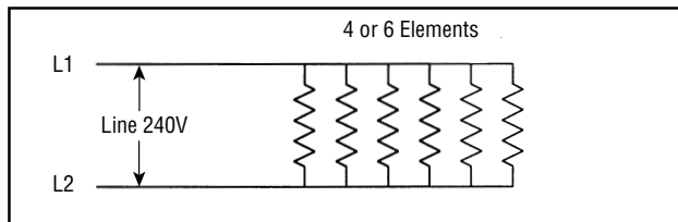
Figure 1 — 240 Volt Heaters
